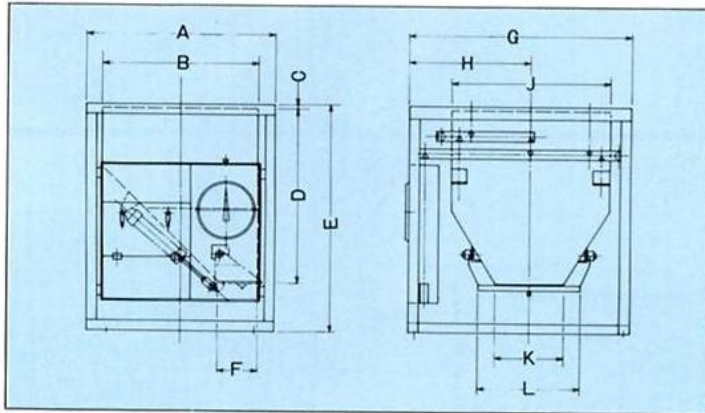
KBS型バッチスケール仕様 (計量物：砂利, 砂)
